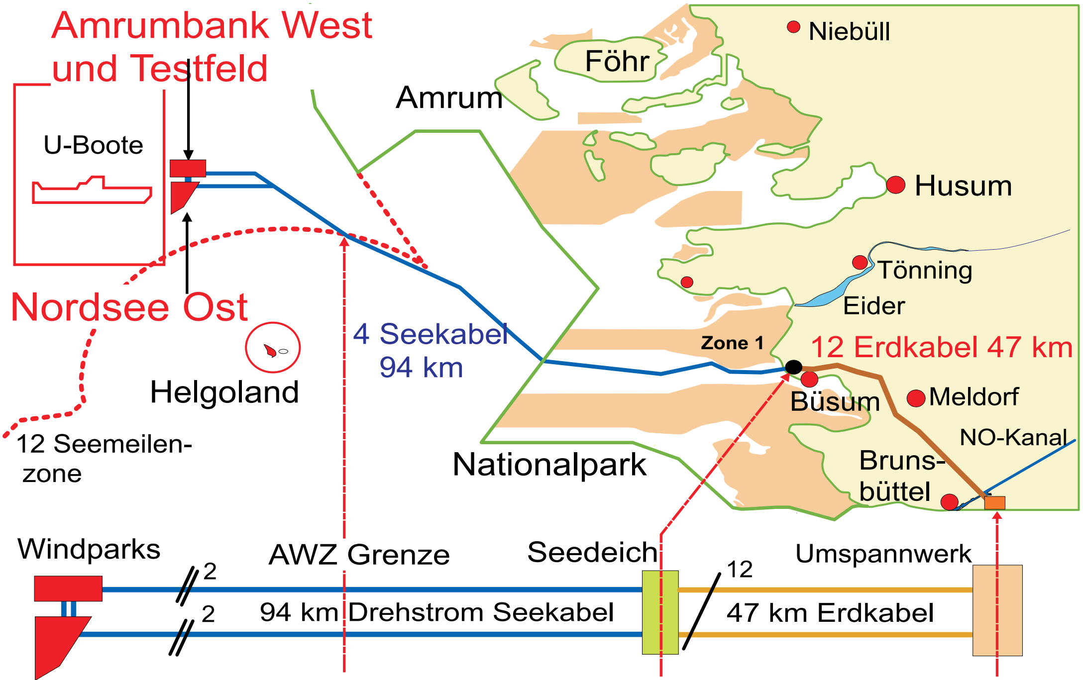
Netzanschlussplanung Helgoländer Cluster
